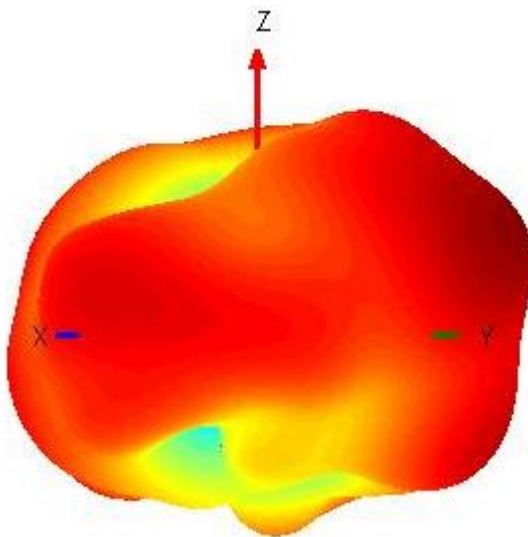
LTE 2170MHZ
