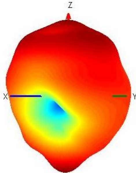
LTE 698MHZ
