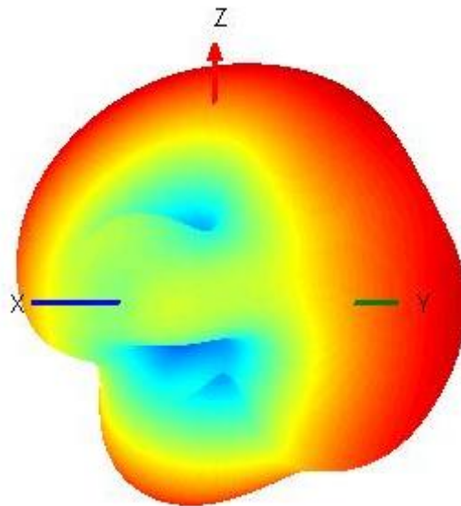
LTE 960MHZ
