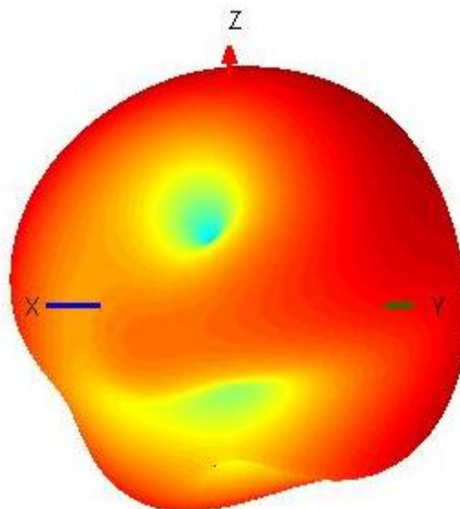
LTE 868MHZ
